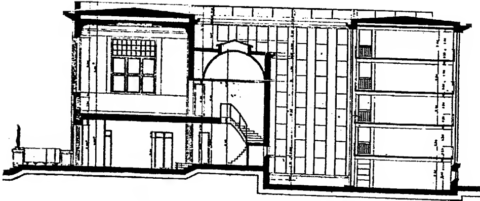
المخطط الداخلي لمبنى المكتبة العامة الحديثة
